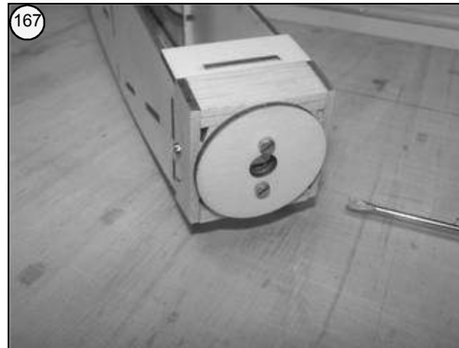
Bilder 167 und 168 - Hilfsspant MT 13 am Motorspant anschrauben und den Rumpfkopf mit Schleifklotz und feinem Schleifpapier verrunden. Hilfsspant MT 13 dient dabei als Schleifanschlag.
