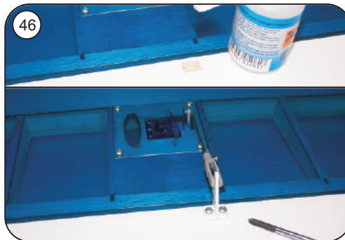
Ruderhorn mit Speedkleber aufsetzen und verschrauben
