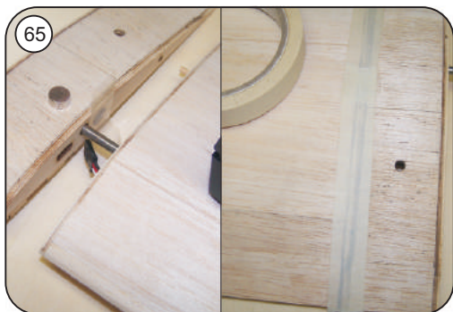
Öffnung für Magnet M 13 von aussen mit Klebestreifen verschliessen, Fläche mit M 15 aufstecken, mit Kreppband fixieren
