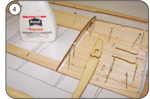
Rippe F 5 einleimen
