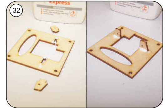
Servohalterung aus F 33 und F 34 herstellen
