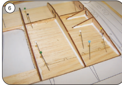
Rippe F 9 einleimen und gerade ausrichten, Klebestellen nachträglich vermuffen
