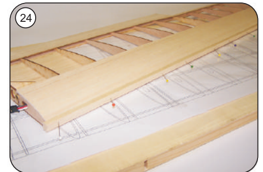
Nasenleiste F 25 ankleben
