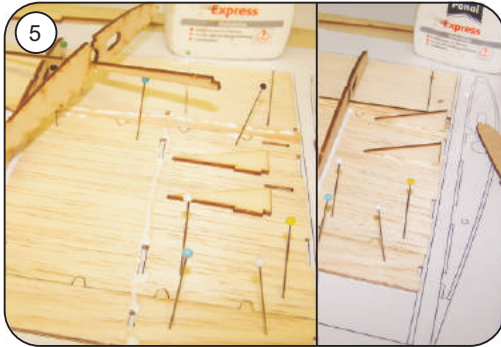
Rippe F 6 mit Formstütze F 7 und Winkelstützen F 8 einleimen
