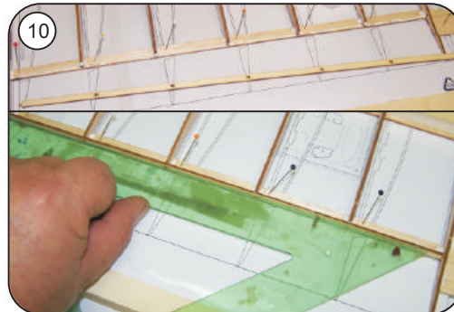
Querruder- Anschlag F 18 einkleben und gerade ausrichten
