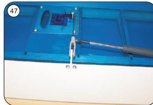
Servo und Querruder in Neutralstellung bringen und mit der Klemmschraube am Gabelkopf sicher fixieren
