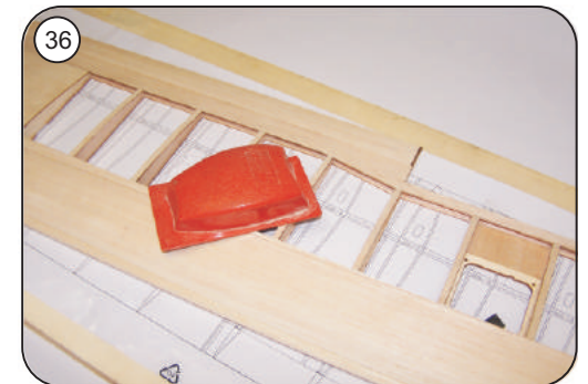
Gesamte Tragfläche sauber verschleifen
