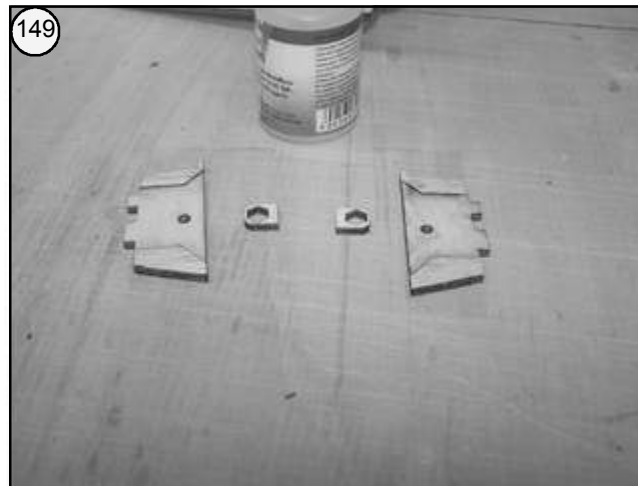
Bild 149 - Füllecken Mt 2 und Mt 3 mit Tesafilm an Mt 1 anheften, mit dünnem Sekundenkleber verkleben.
