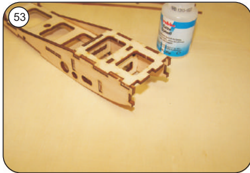
Boden unten M 5 einsetzen und anheften
