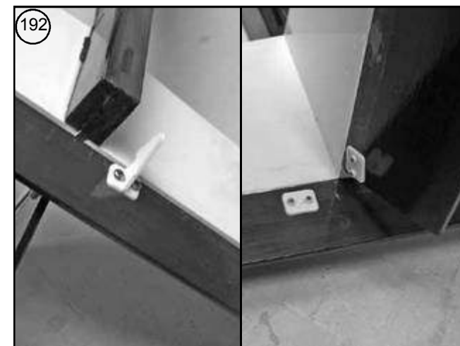
Bild 192 - Ruderhorn am Höhenruder anschrauben.
