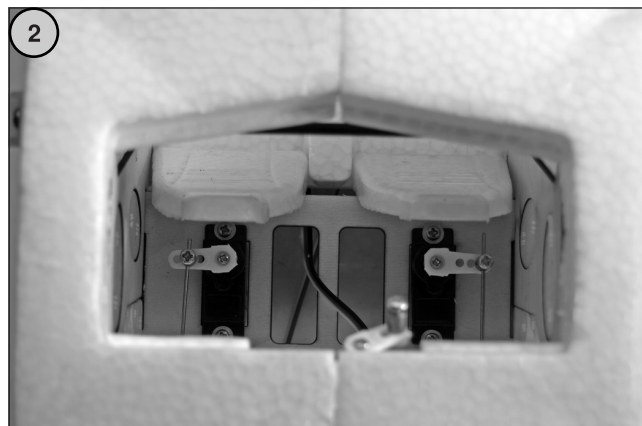
Bild 2 - Falls erforderlich, das Höhenrudergestänge an der Kupplung des Höhenruderservos lösen.
