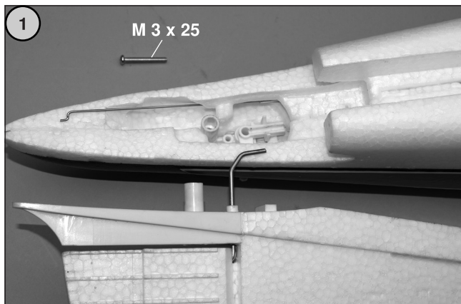
Bild 1 - Die Anlenkungen von Höhen- und Seitenruder im Rumpfeinde.
