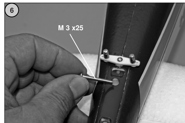
Bilder 6 und 7 - Höhen- und Seitenleitwerk am Rumpfeinde verschrauben.
